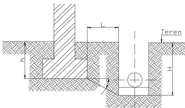
Obrázek 1: Bezpečná vzdálenost dna výkopu od budovy
