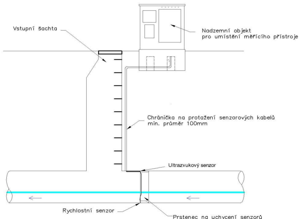
Obrázek 2: Schéma měrného objektu na stoce (Typický měrný profil)
