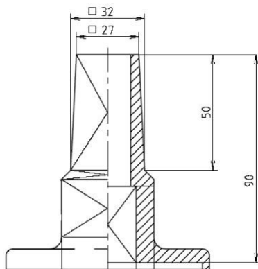
Obrázek 3: Ovládací prvek – zakončení vřetene čtyřhranem
